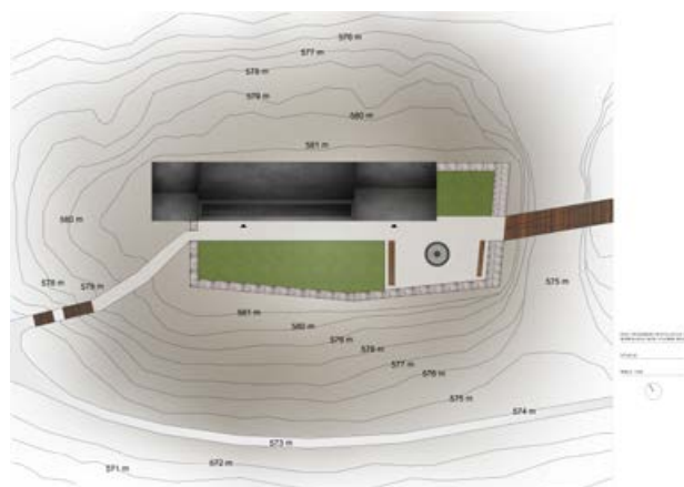
Situacijski prikaz grajskega jedra
