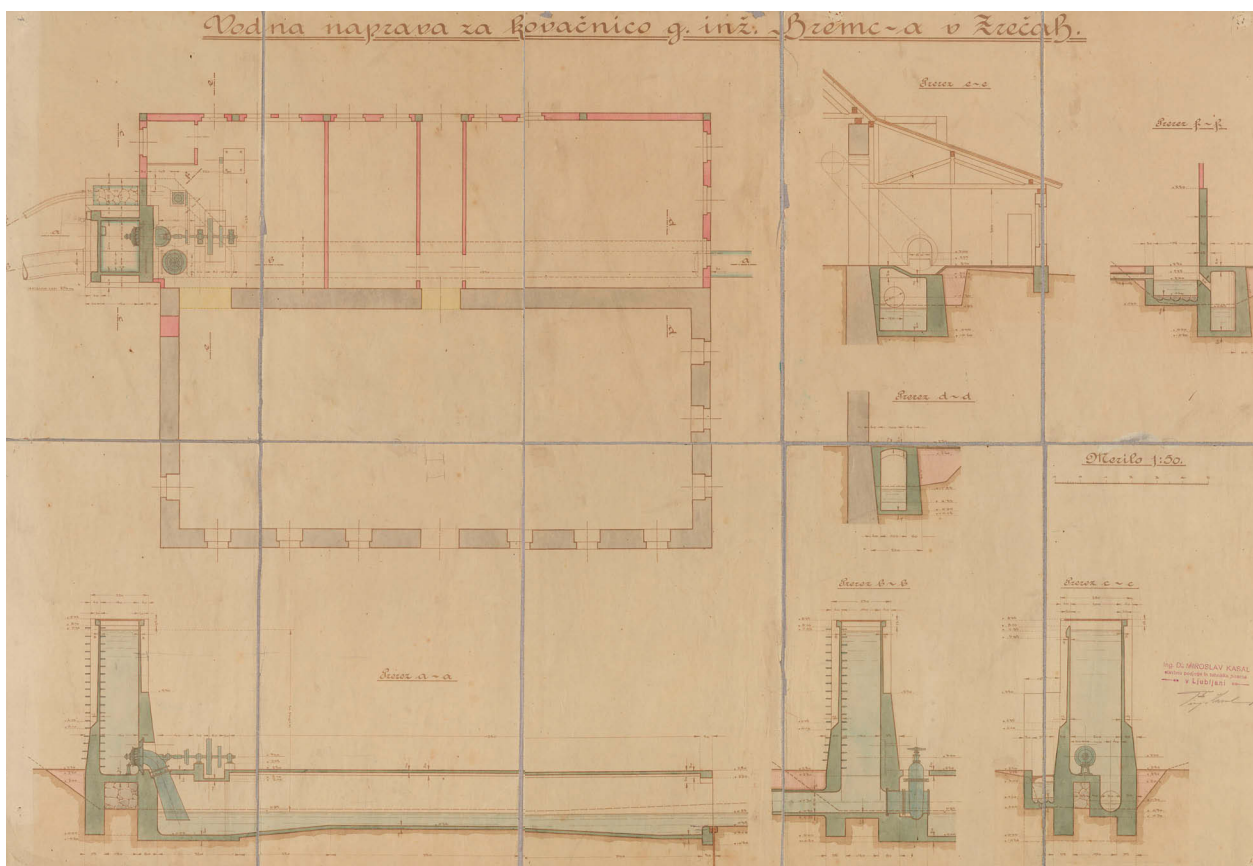
Slika 3: Načrti inž. Miroslava Kasala in Milka Bremca za kovačijo (vir: Arhiv Republike Slovenije, fond: SI AS Milko Bremec (Melhior), 1890–1986, šk. 16).
