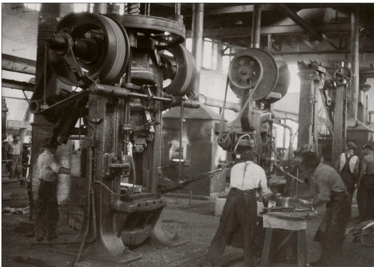
Slika 5: Pogled na zreško kovačijo s stroji v letih pred drugo svetovno vojno (vir: SI AS 1225 Milko Bremec (Melhior), 1890–1986, šk. 32).
