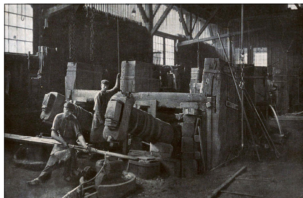
Slika 18: Fotografija vodno gnanega kovaškega kladiva repača, imenovanega tudi norec ali tolkač (vir: SI 1225 Milko Bremec (Melhior), 1890–1986, šk. 32).
